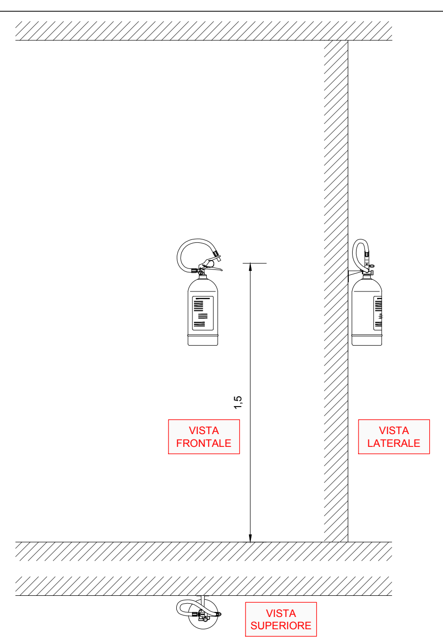
PARTICOLARE INSTALLAZIONE ESTINTORE - SCALA 1:20
