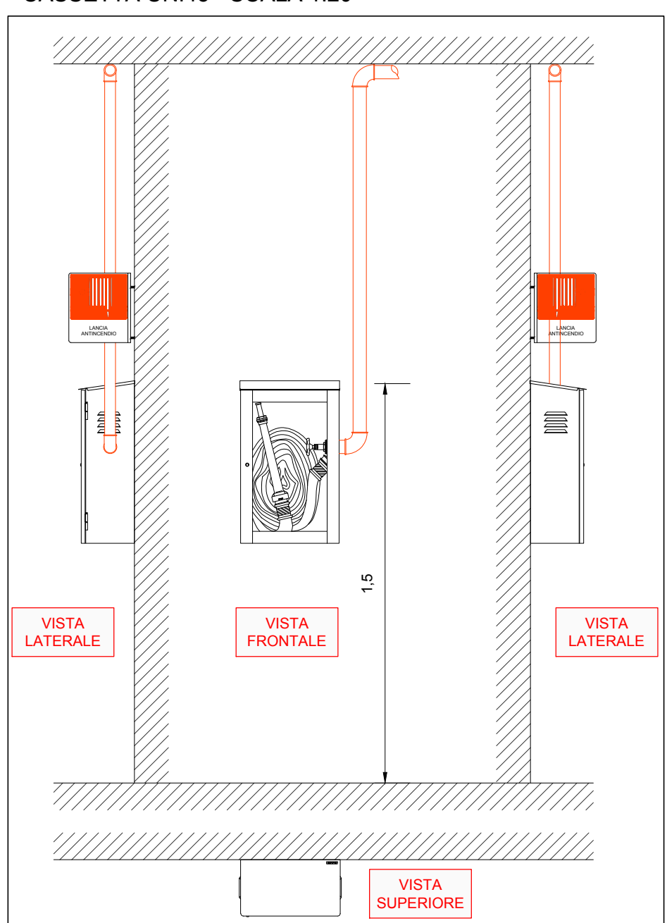
PARTICOLARE INSTALLAZIONE CASSETTA UNI45 - SCALA 1:20
