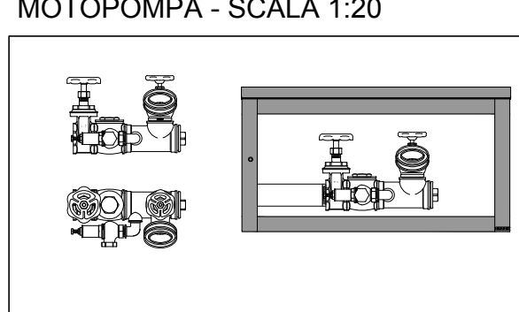
PARTICOLARE CASSETTA ATTACCO MOTOPOMPA - SCALA 1:20
